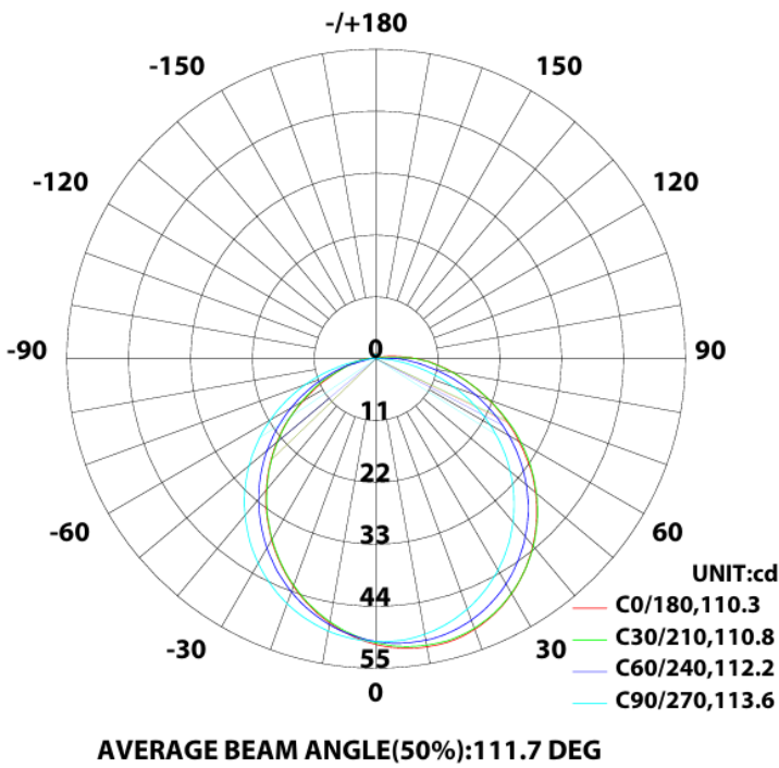
Diagramme de distribution de l'intensité lumineuse
