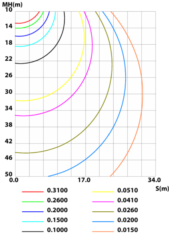
Diagramme isolux dans le plan
