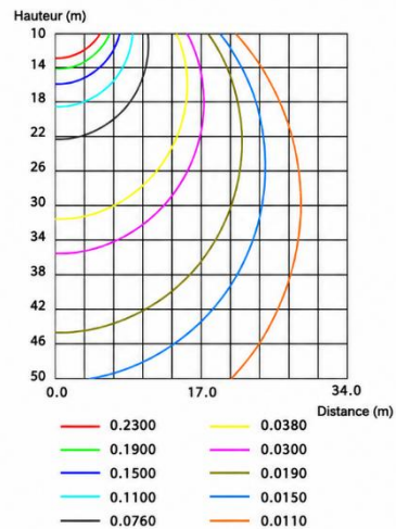
DIAGRAMME ISOLUX DU PLAN C0 (UNITÉ: lx)
