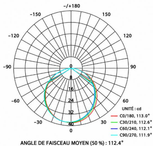
DIAGRAMME DE DISTRIBUTION DE L'INTENSITÉ LUMINEUSE
