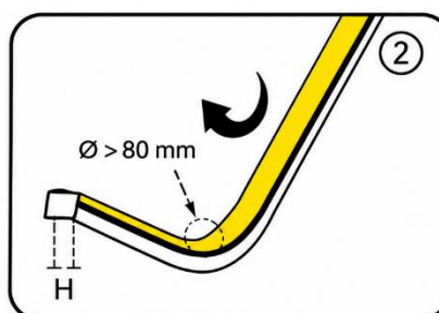
2. Série de pliage supérieur Sens correct de pliage
