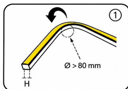
1. Série de pliage supérieur Sens correct de pliage
